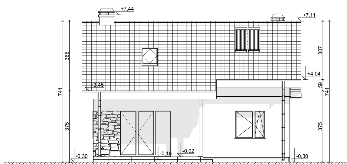
ELEWACJA OGRODOWA
